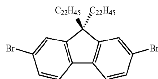
F22-dibromide
